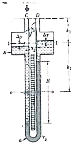
Fig.(2.9) Micromanometer
