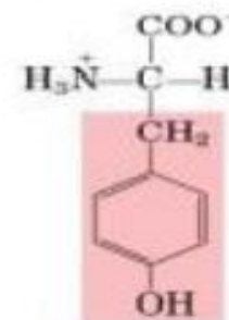
Tyrosine
