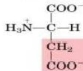
Aspartate
