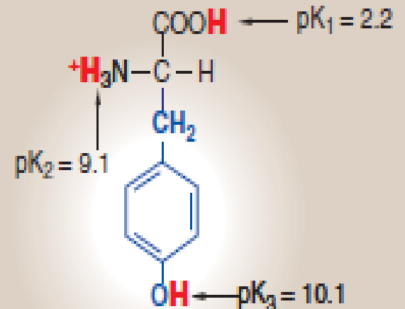
Tyrosine
